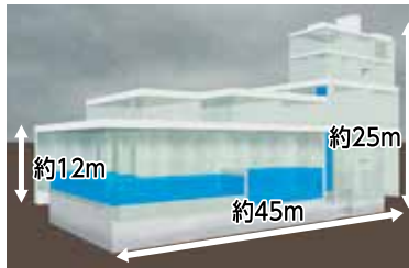
雨水貯留施設 貯留量:約4,000m 3
